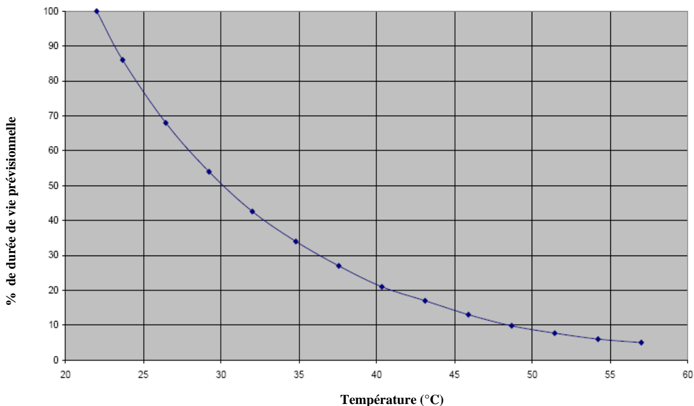
Caractéristiques de durée de vie en fonction de la température
